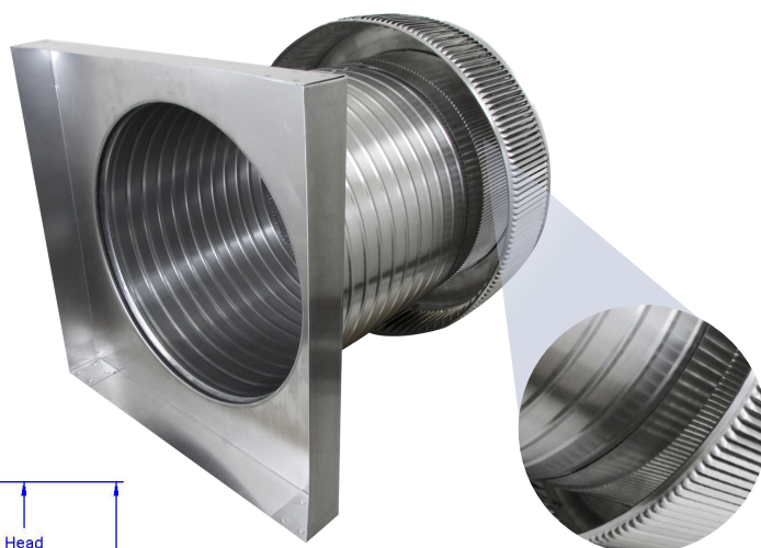
Inside Louvers
