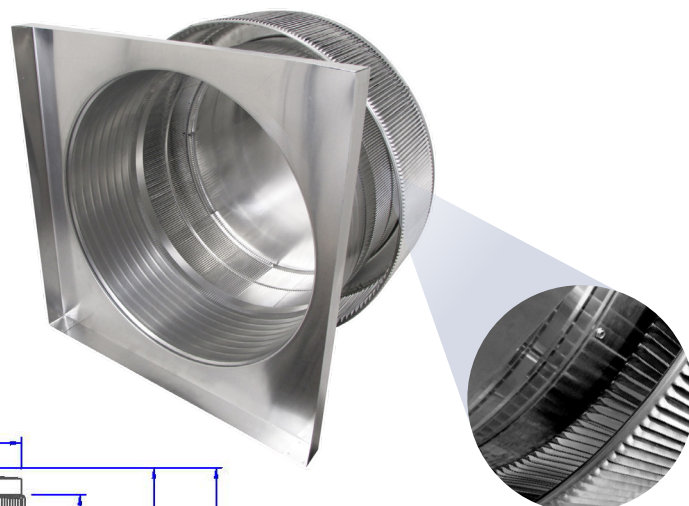
Inside Louvers
