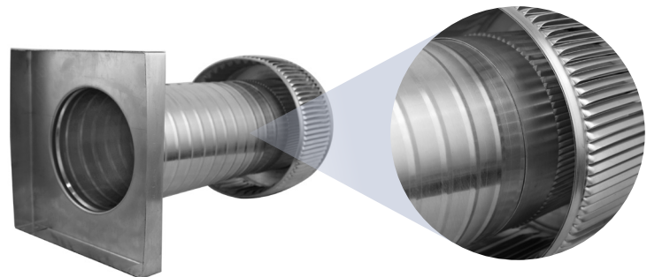
Inside Louvers
