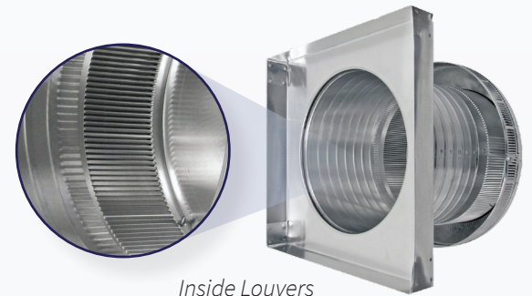
Inside Louvers
